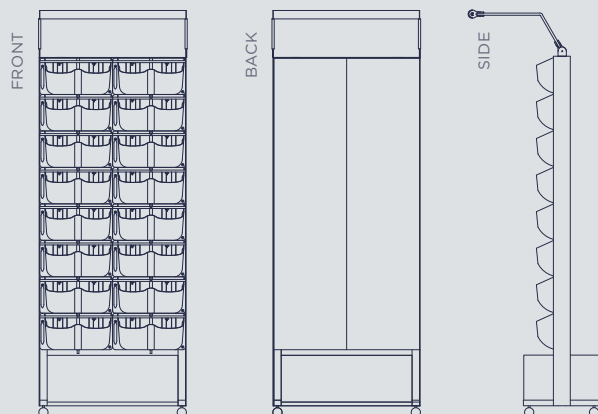
Model: S2-8 78W x 217H x 40D cm - podwójne moduły roślinne - 32 roślin - jednostronny roślinnie - panele akustyczne z tyłu
