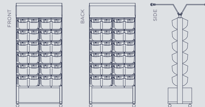
Model: S2-6-2 78W x 177H x 40D cm - podwójne moduły roślinne - 48 roślin - dwustronny roślinnie
