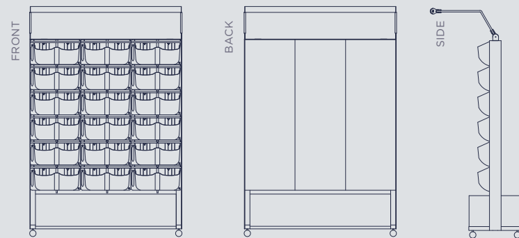
Model: S3-6 117W x 177H x 40D cm - podwójne moduły roślinne - 36 roślin - jednostronny roślinnie - panele akustyczne z tyłu
