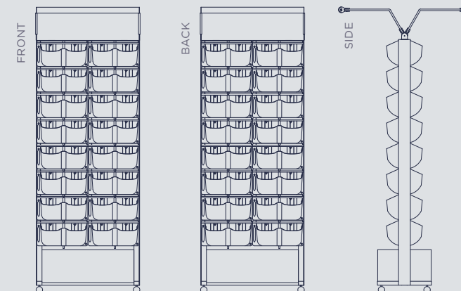
Model: S2-8-2 78W x 217H x 40D cm - podwójne moduły roślinne - 64 roślin - dwustronny roślinnie
