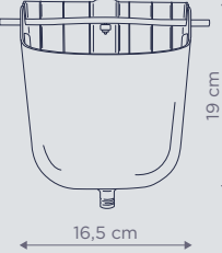
Moduł pojedynczy na roślinę 4Nature System Indeks: P13739632
