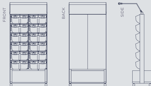
Model: S2-6 78W x 177H x 40D cm - podwójne moduły roślinne - 24 roślin - jednostronny roślinnie - panele akustyczne z tyłu
